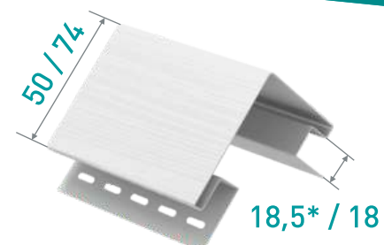
Наружный угол 50 / 74 мм
